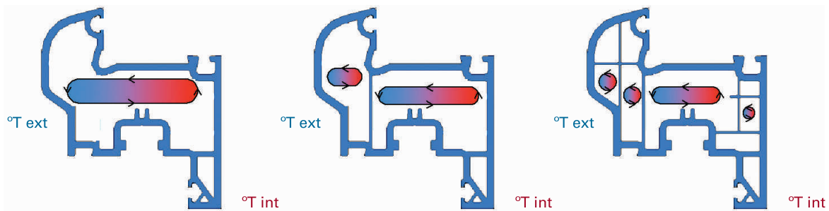
Situación de invierno ( ^{\circ}T_{ext} < ^{\circ}T_{int} )
