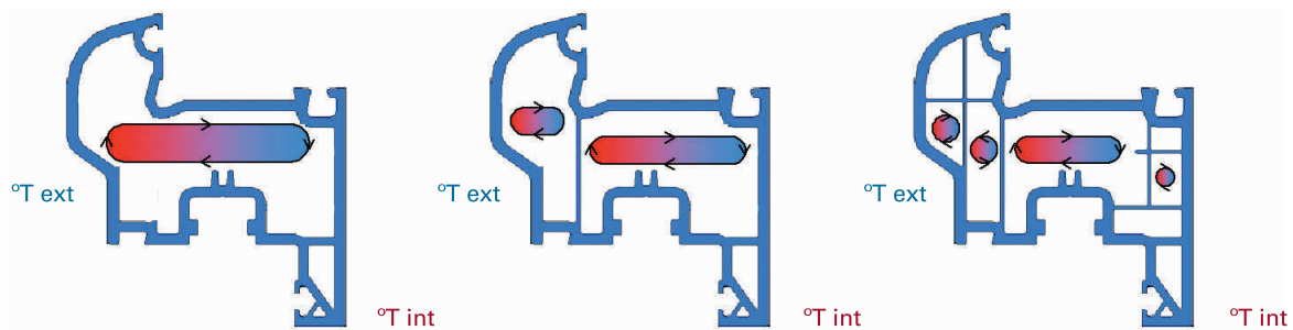
Situación de verano ( ^{\circ}T_{ext} > ^{\circ}T_{int} )
